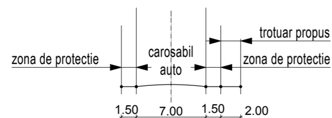
STRAZI DE CATEGORIA A-III-A CU 2 BENZI DE CIRCULATIE
